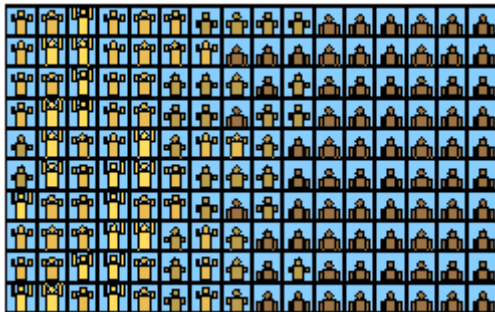
La ola :Tamas Vicsek
